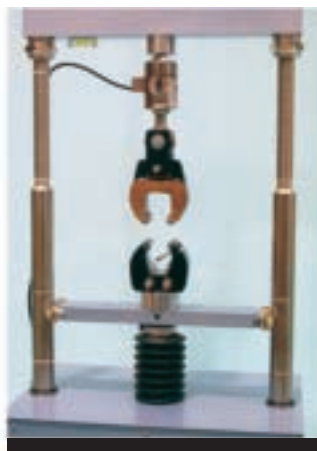
Растяжение растворных брикетов
